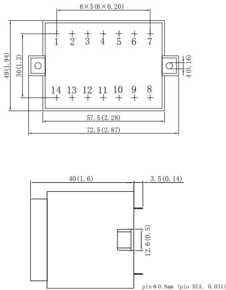
Esquemático
