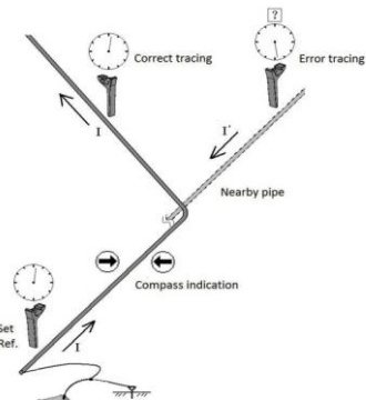
Fig.4.6Intelligent tracing demo.
